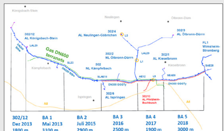
Bild 1: Streckenprofil des Bauprojektes Kämpfelbach mit den jeweiligen Bauabschnitten [6]
